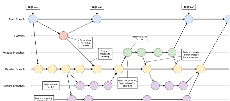
Figura 1: struttura dei branch all'interno della repository
